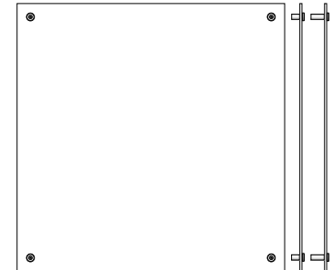
kit 110 V (kit A 30 / kit A 50) w 1000 x h 1000 x d 8mm w 39,37 x h 39,37 x d 0,31"
