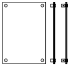
kit VV A3 (kit C 15 / kit D 15) [w 297 x h 420 x d 4mm] x 2 [w 11,69 x h 16,54 x d 0,16"] x 2
