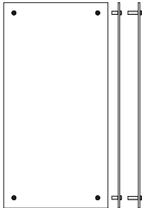
kit 109 V (kit B 30 / kit B 50) w 500 x h 1000 x d 8mm w 39,37 x h 11,8 x d 0,31"
