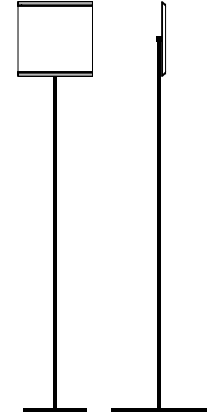
pil 904 P w 210 x h 1155 x d 270 mm (pil 204 P : w 210 x h 210 x d 11 mm) w 8,27 x h 45,47 x d 10,63\"/> (pil 204 P : w 8,27 x h 8,27 x d 0,43\"/>
